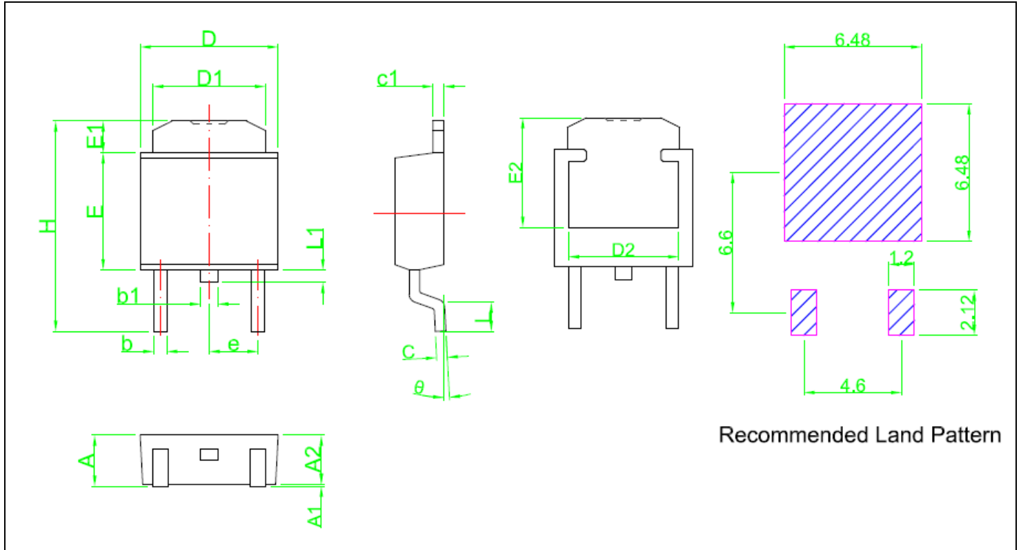
原尺寸圖
